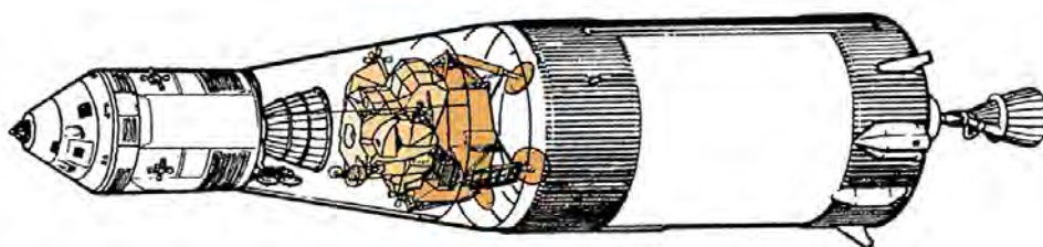
Schéma de l'ensemble du 3 e étage de la fusée Saturne V en orbite autour de la Terre.
