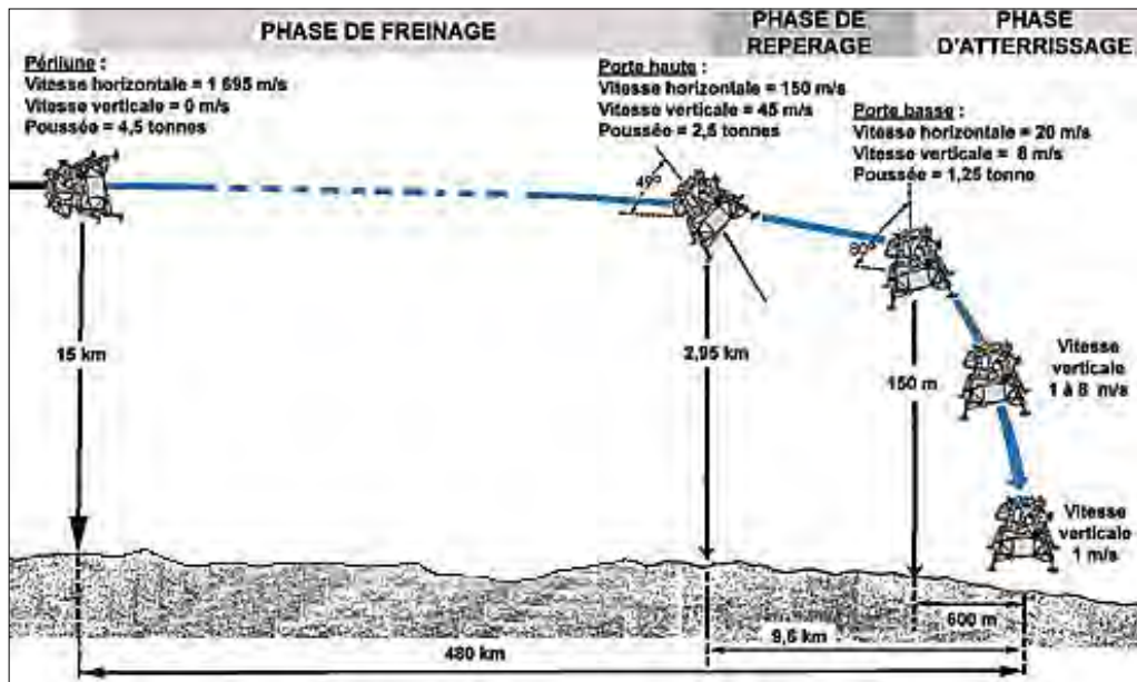
Schéma de la navigation et de l'alunissage du module lunaire.
