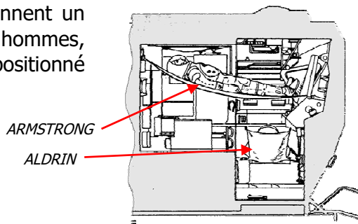
Schéma d'installation des 2 astronautes
