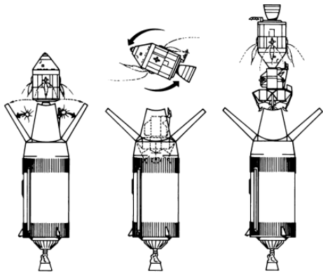
Schéma du retournement et d'arrimage des différents modules.
