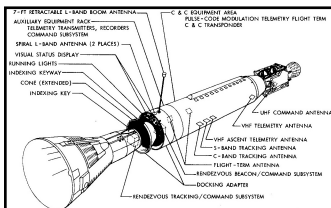
Schéma d'amarrage GÉMINI/AGÉNA
